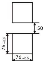
开孔尺寸
