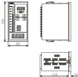
外形尺寸
