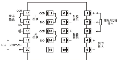
接线端子图
