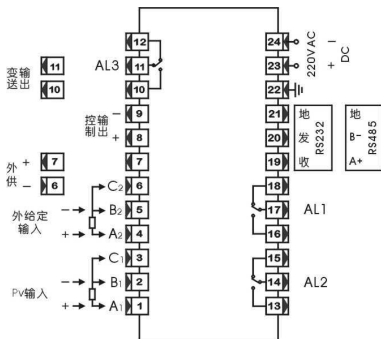
接线端子图
