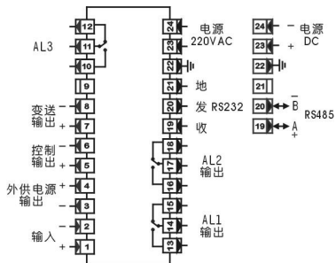
接线端子图
