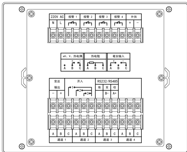
图 2.3.1.1 后端子图
